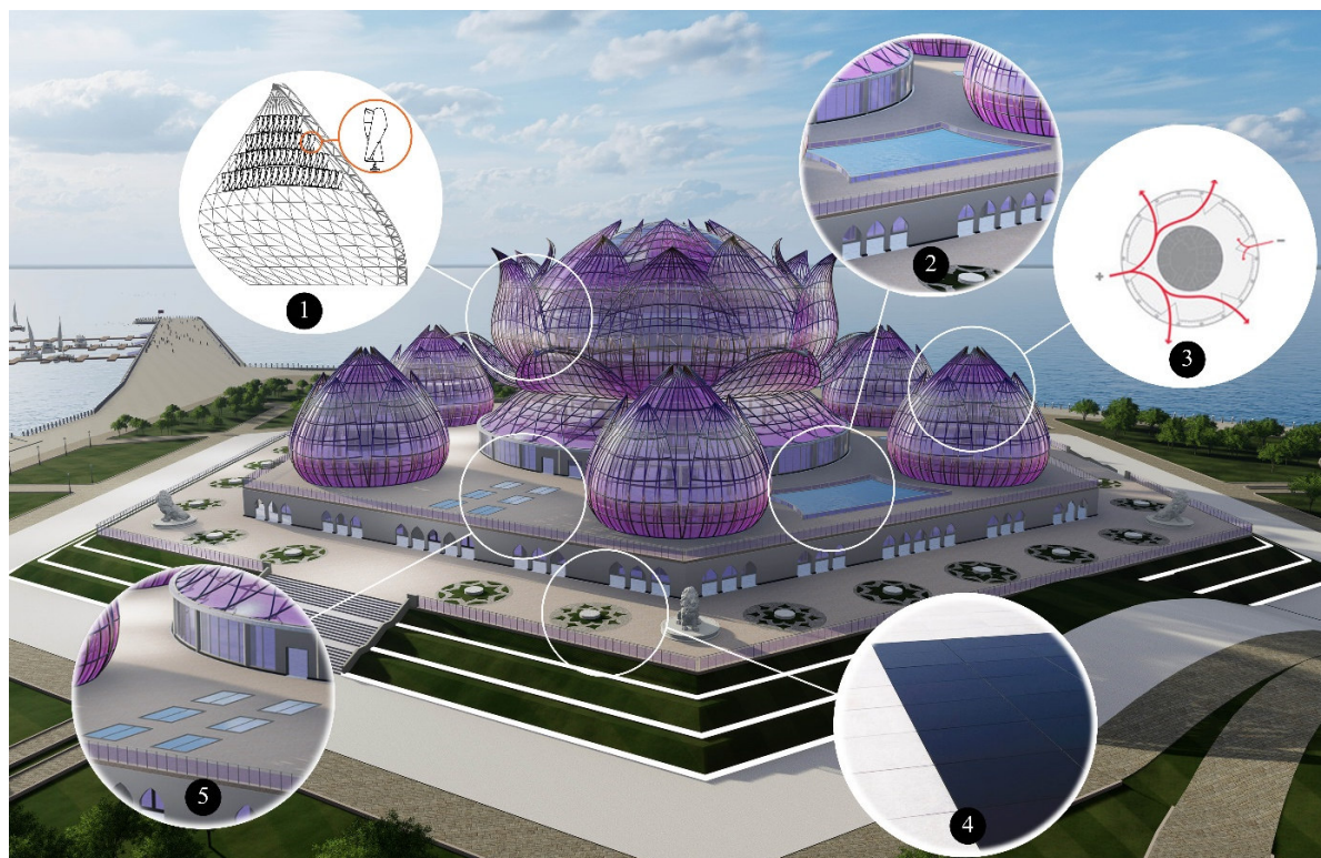
Рис. 19. Национальный общественный центр в Шри-Ланке: 1 – применение ветряных турбин в лепестках цветов, 2 – использование дождевой воды в пруда, 3 – естественная вентиляция с двойным фасадом, 4 – использование прогулочных солнечных панелей, 5 – оптимизация системы дневного освещения
