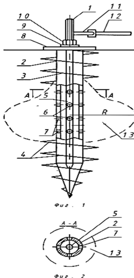
Рис. 1. Конструкция винтовой сваи Приняты следующие обозначения: 1 – хвостовик под патрон бурового вращателя; 2 – полая (цилиндрическая) центральная труба; 3 – верхний конусный шнек по трубе; 4 – нижний конусный шнек; 5 – внутренняя трубка; 6 – отверстия для выхода твердеющего раствора во внутренней трубке; 7 – отверстие во внешней трубе; 8 – пакер над шнеком; 9 – шайба; 10 – гайка прижимная; 11 – патрубок-штуцер для шланга насоса; 12 – нагнетательный шланг; 13 – массив грунта; R – радиус закрепления грунта
