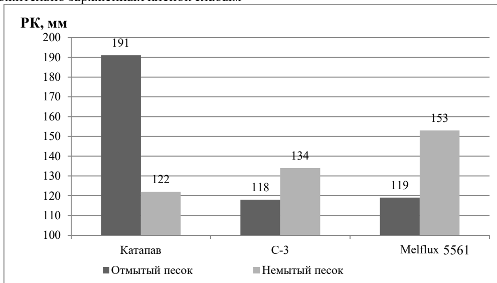
Рис. 2. Эффективность действия катион- и анионных разжижителей после отмывки пленок на кварцевом песке соляной кислотой
