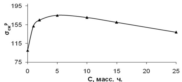
Рис. 5. Зависимость \sigma_{сжT} и \sigma_{сжP} от концентрации Al_2O_3 . Образцы отверждены по режиму II
