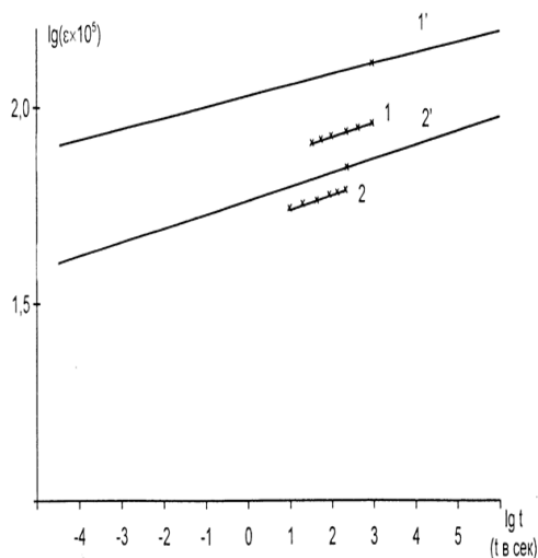
Рис. 3. График изменения относительных деформаций образцов в зависимости от длительности их испытаний (в логарифмических координатах). Опытные значения деформаций при R = 0,8R_{пр} : 1 – для керамзитобетона; 2 – для тяжелого бетона. Расчетные значения разрушающих деформаций: 1' – для керамзитобетона; 2' – для тяжелого бетона
