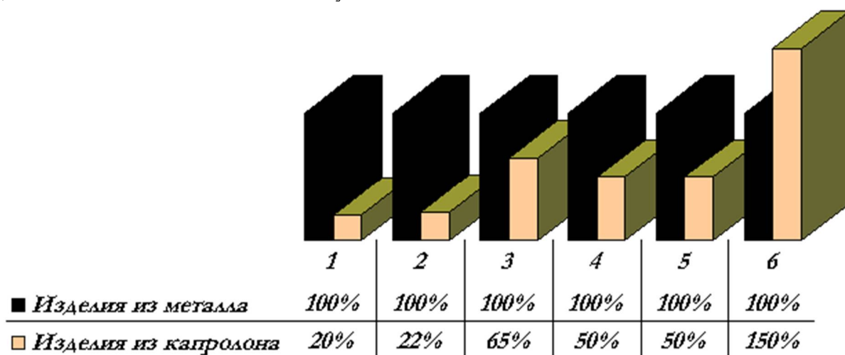
Рис. 1. Эффективность капролона по сравнению с металлом
