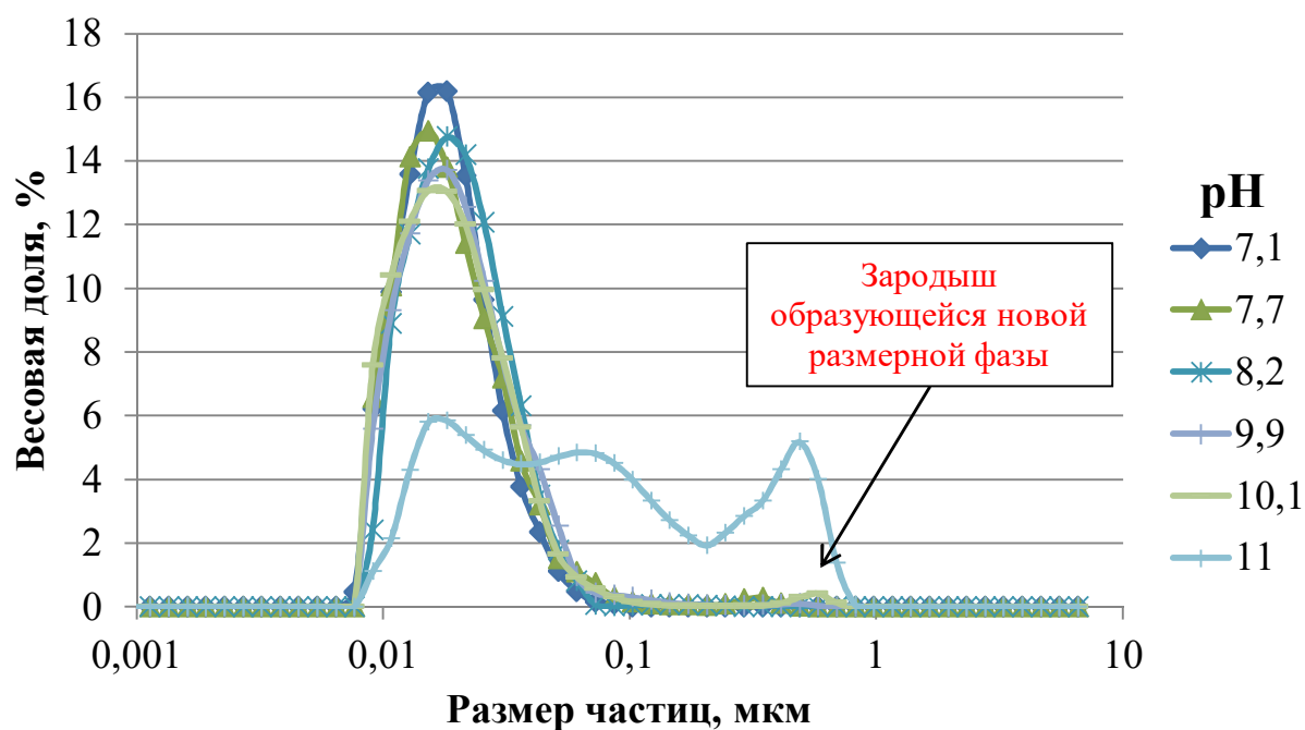
Рис. 3. График распределение размеров НЧС раствора AgВiон-2 в зависимости от pH среды
