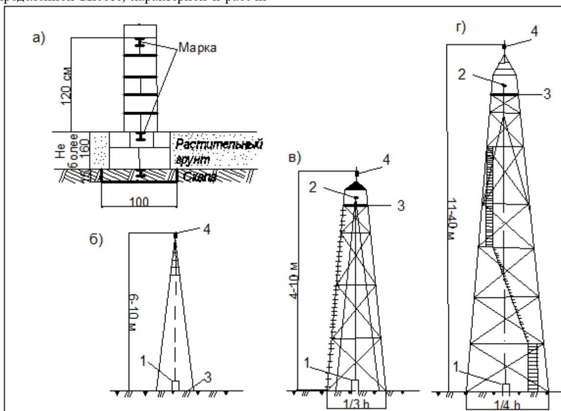
Рис. 1. Геодезические знаки:
