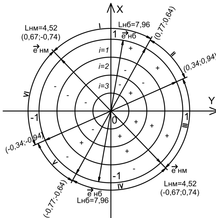
Рис. 2. Наибольшее и наименьшее значения интенсивности трещиноватости Лебединского месторождения: I, II, ..., VI – номера секторов направлений единичного круга; L_{НБ}=7,96 – наибольшее, L_{НМ}=4,52 – наименьшее значения интенсивности трещиноватости. \vec{e}_{НБ} , \vec{e}_{НМ} – направления, по которым достигаются соответственно наибольшее и наименьшее значения
