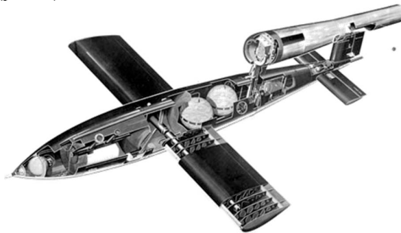
Рис. 3. Самолет - снаряд Фау-1
