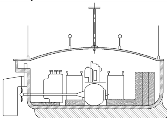
Рис. 1. Дистанционно управляемый кораблик Н. Теслы
