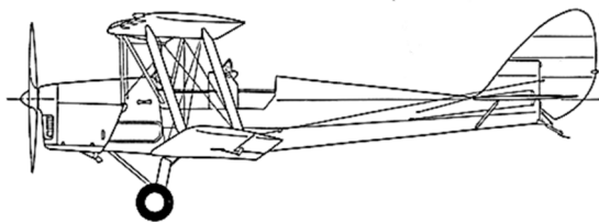
Рис. 2. БПЛА – мишень DH.82B Queen Bee
