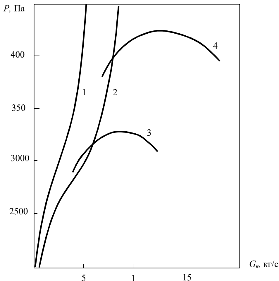
Рис. 3. Характеристики аспирационного тракта (1 – без подсосов, 2 – с подсосами, F = 0,076 ) и вентиляторов (3 – Д-12, n = 970 об/мин, t = 75 °С, 4 – Д-15,5, n = 970 об/мин, t = 77 °С)
