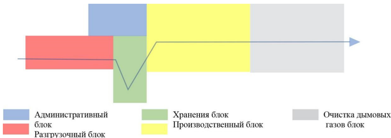
Рис. 2. Технологический процесс производства и зонирование мусоросжигательной электростанции
