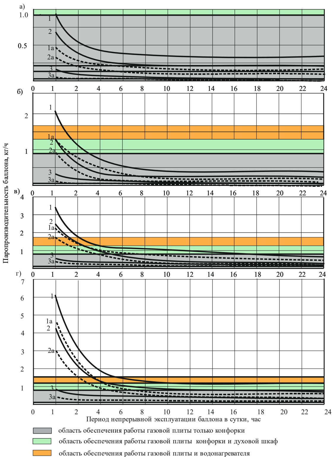
Рис. 1. Паропроизводительность композитных баллонов вместимостью: а) 5 л; б) 12,7 л; в) 24,5 л; г) 47 л при периодическом использовании газа:
