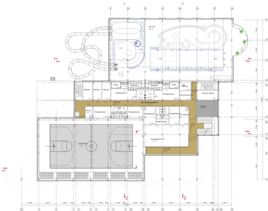
Рис. 4. План 2 этажа спортивно-оздоровительного комплекса «Флагман»
