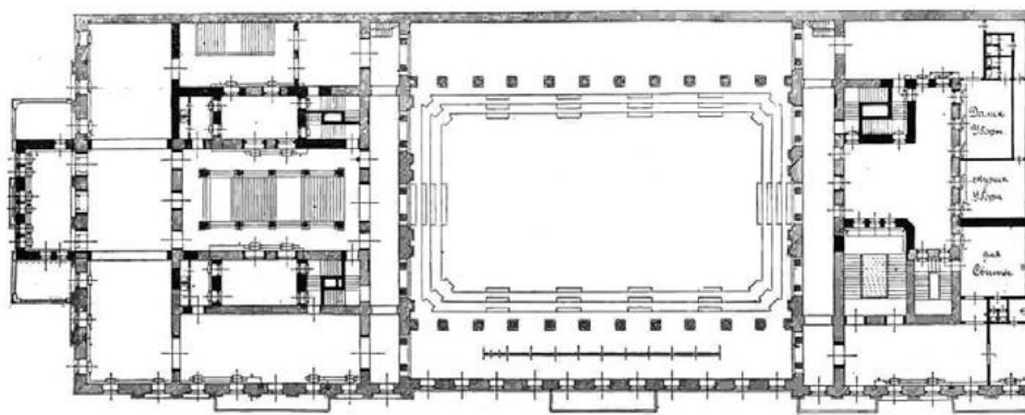
193. Планъ 2-го этажа.
