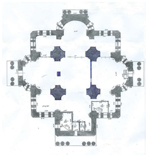
Рис. 5. План храма
