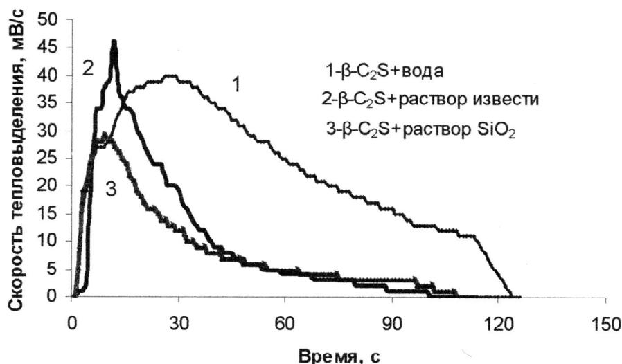
Рис. 3. Скорость тепловыделения при гидратации \beta - C_2S
