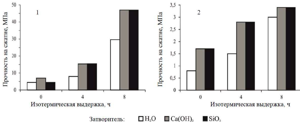
Рис. 4. Прочность на сжатие белитовых фаз в автоклавных условиях (1 – \beta - C_2S , 2 – \gamma - C_2S )
