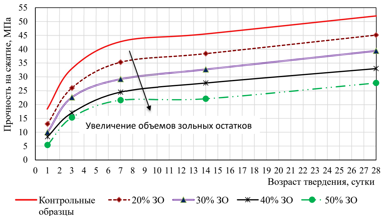
Рис. 6. Влияние замены части вяжущего золными остатками ТЭС Вунг Анг на прочность цементно-песчаного камня на сжатие
