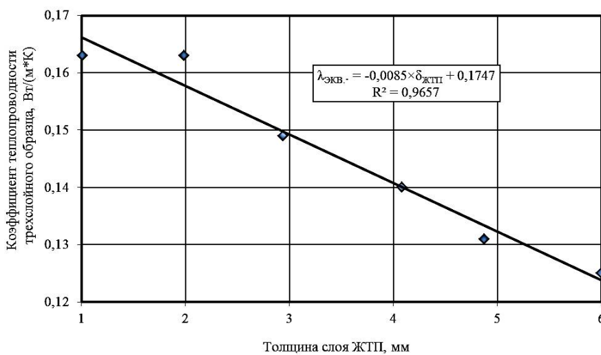
Рис. 3. Изменение эквивалентного коэффициента теплопроводности трехслойного образца в зависимости от толщины слоя ЖТП
