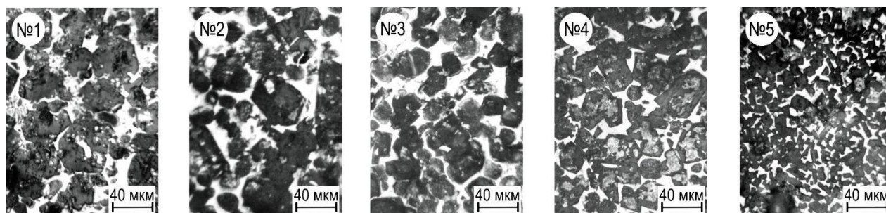
Рис. 1. Изменение микроструктуры клинкера в зависимости от положения зоны спекания и КПД холодильника
