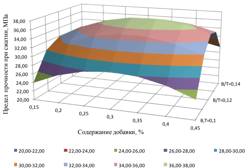
Рис. 3. Зависимость прочности прессованных гипсовых образцов от содержания добавки поливинилового спирта и водотвердого отношения
