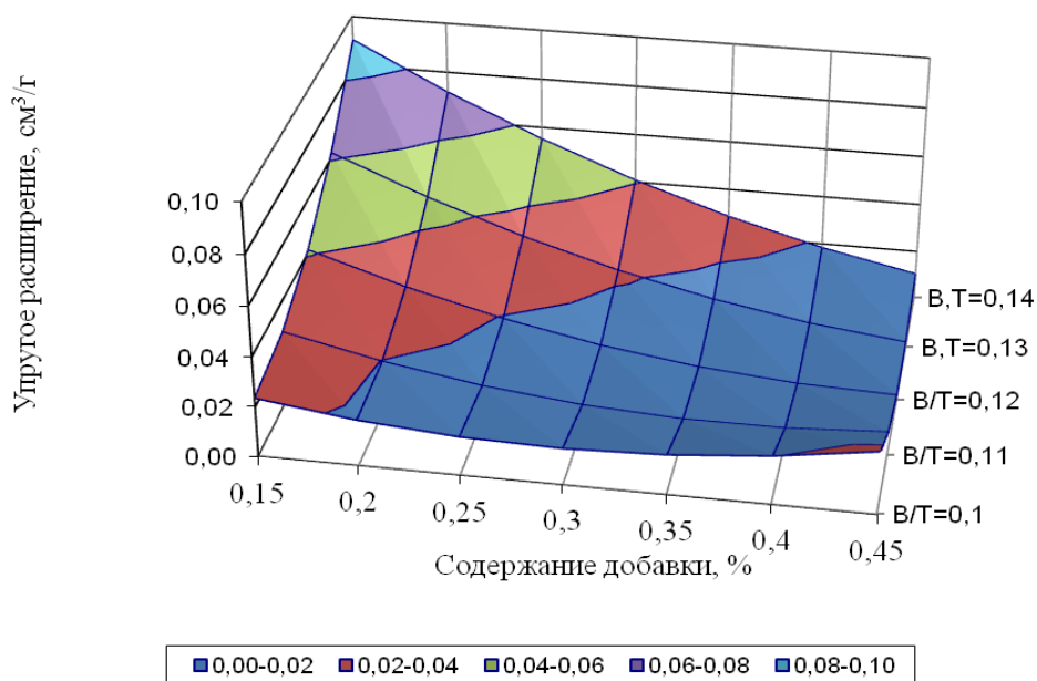
Рис. 2. Зависимость упругого расширения гипсовых образцов от добавки поливинилового спирта
