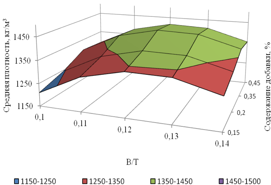
Рис. 1. Зависимость средней плотности от содержания добавки поливинилового спирта и водотвердого отношения
